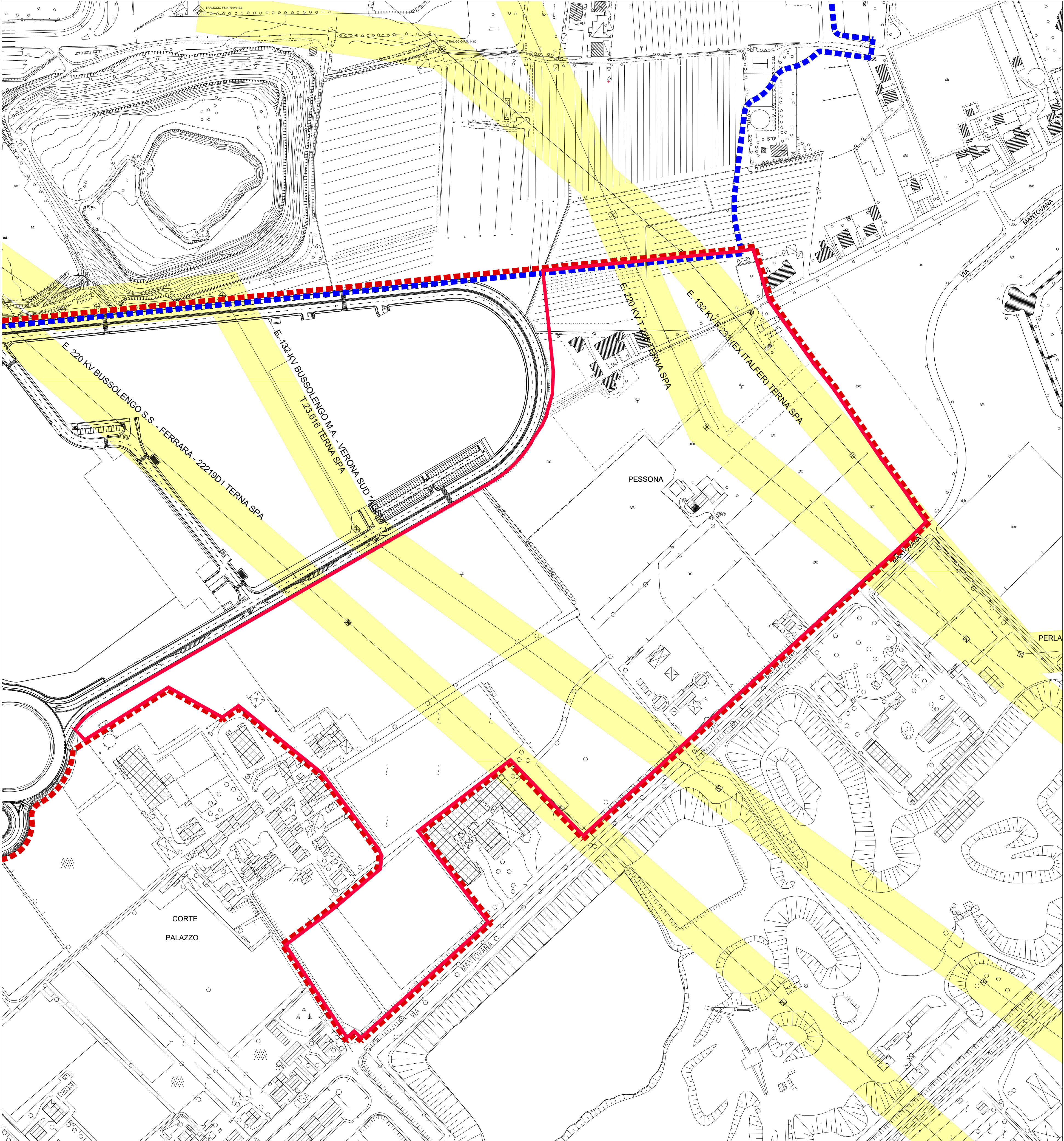
DETTAGLIO FASCE DI RISPETTO DEGLI ELETTRODOTTI SCALA 1:2.000
